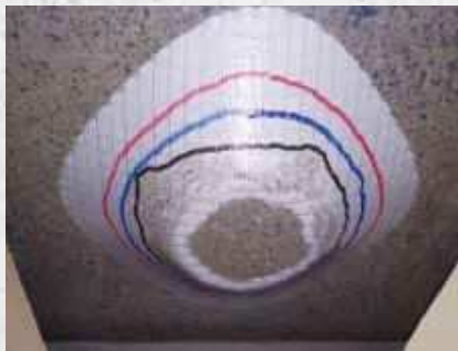
押抜き試験状況 (V2仕様)
