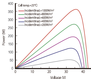
放射照度特性 (P-V) : LR4-60HPH-365M
