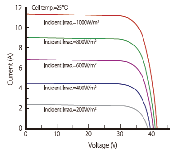
放射照度特性 (I-V) : LR4-60HPH-365M
