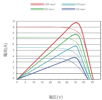
電流電圧・電力電圧特性曲線 (310W)
