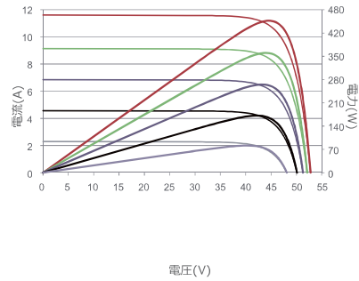
I-V 特性曲線 (455W)
