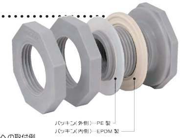
容器側面への取付例 PE フィッティング + プラグ
