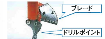
ドリルポイントブレード
