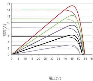
電流電圧・電力電圧特性曲線 (600W)
