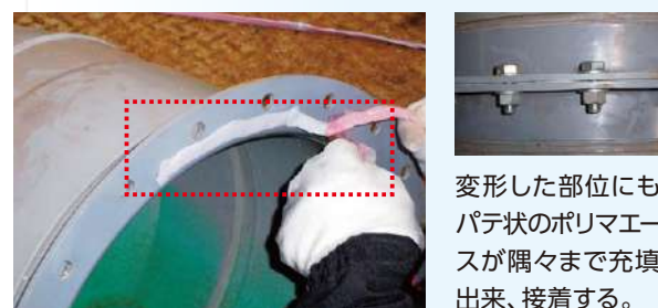
U字ピット内太管で自己融着テープ使用不可の狭小現場で採用
