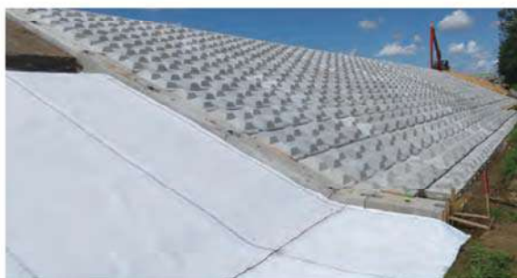
河川護岸(川裏) ブロック敷設状況
