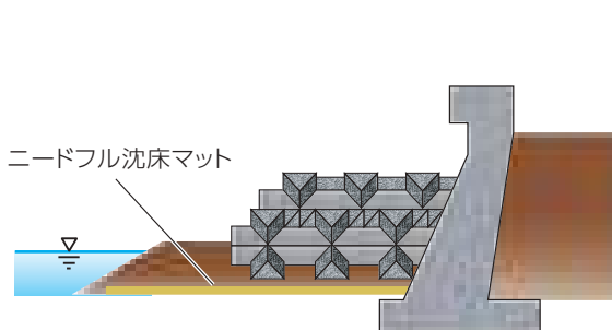
消波ブロック根固工
