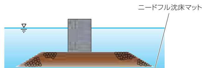
防波堤等の洗掘防止工
