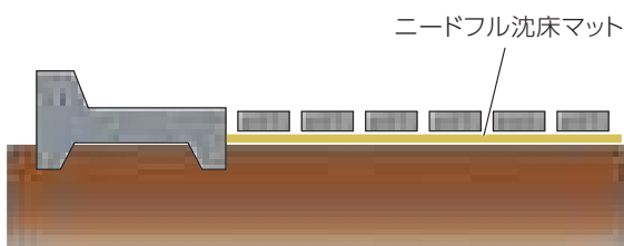
河川護床工
