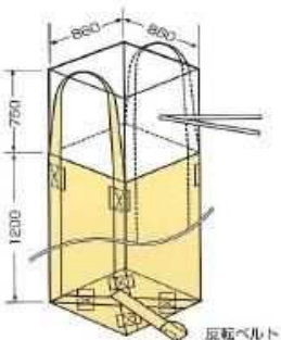
KB-1 角型
